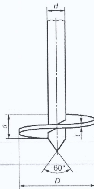
Рисунок Б.1 — Конструкция винтового штампа
