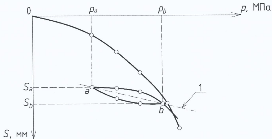
Рисунок Д.1 — График S = f(p) испытания грунта штампом
